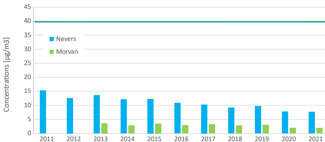
Moyennes annuelles en NO 2 sur le département
