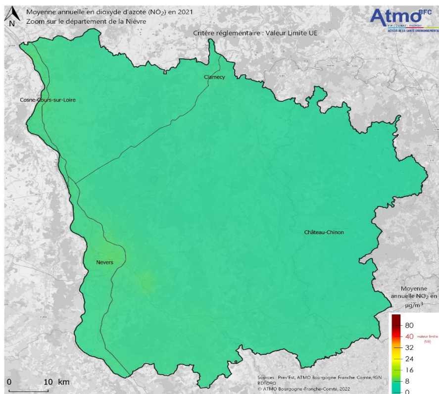
Moyennes annuelles en NO 2 sur le département
