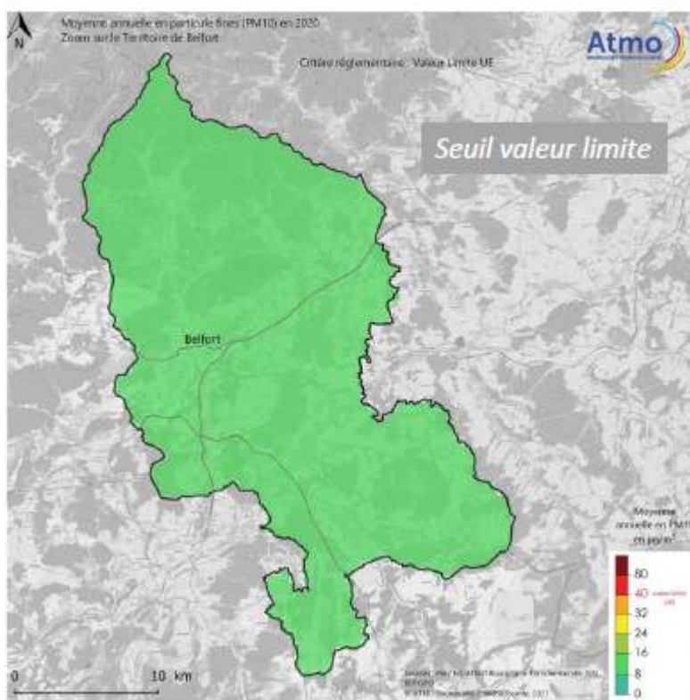
Modélisation sur le territoire de Belfort des PM10 pour l'année 2020
