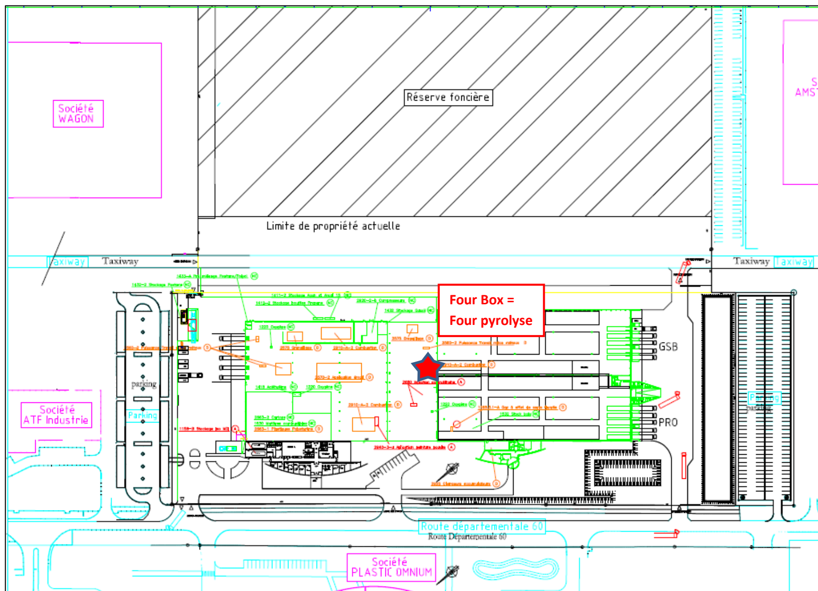
Ce plan permet de localiser l'implantation du « Four pyrolyse » objet du présent dossier.
