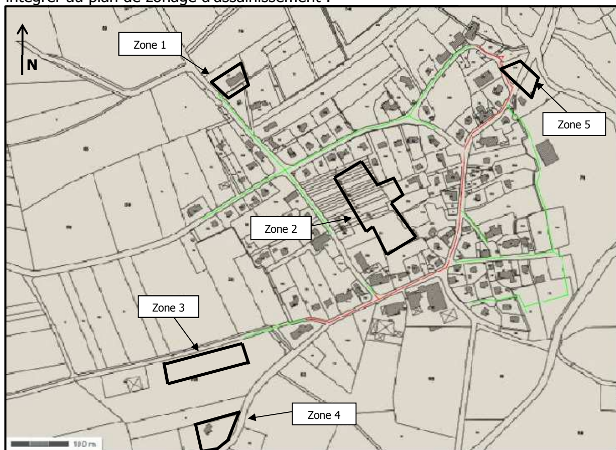
FIGURE 3 - TRACE DES RESEAUX D'ASSAINISSEMENT EXISTANTS + PROJETES
