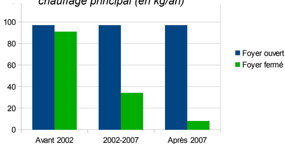
Emissions moyennes annuelles de particules d'un foyer utilisé comme chauffage principal (en kg/an)
