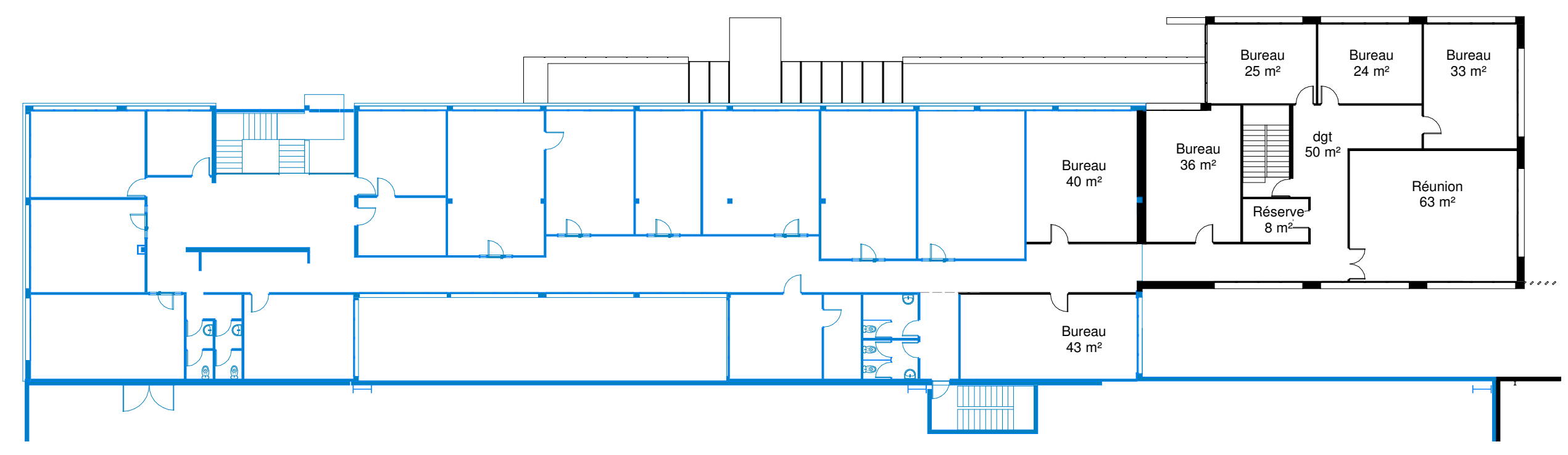
Etage bureaux 1 : 250
