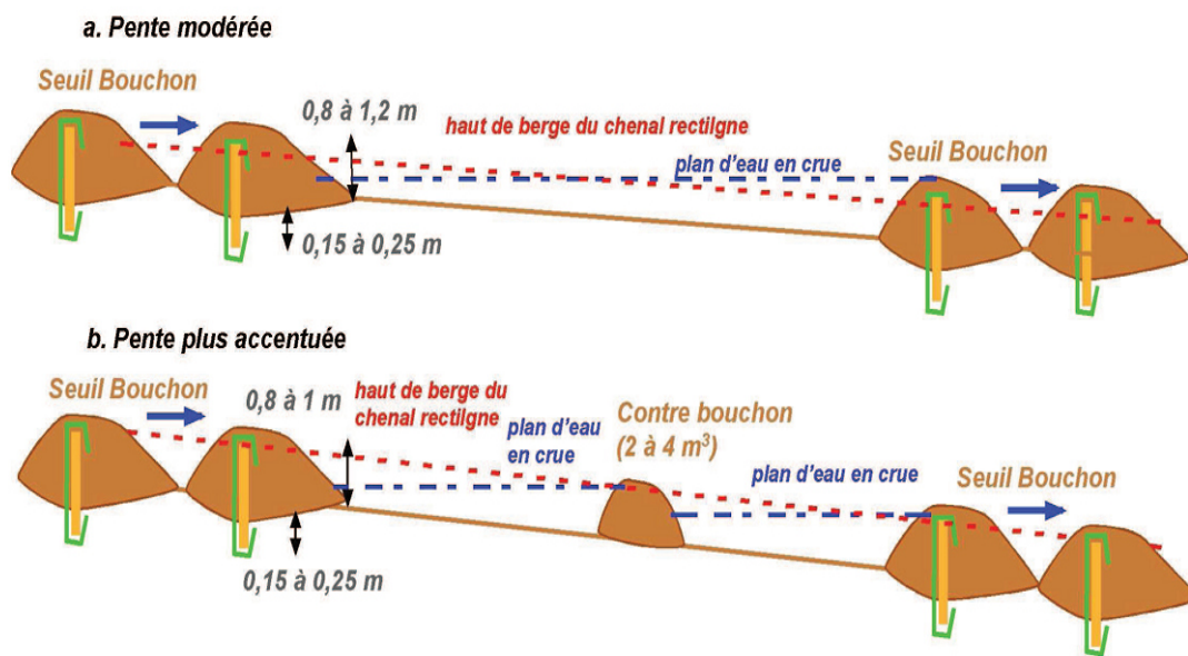
Figure 20. Etagement vertical des bouchons successifs de façon à garantir le recouvrement vertical des plans d'eau induits.
