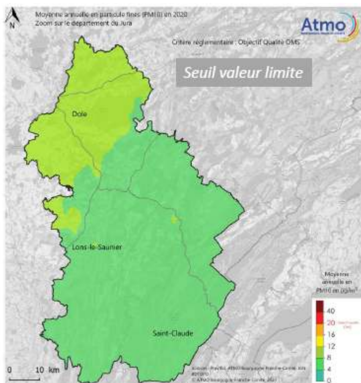
Modélisation sur le Jura des PM10 pour l'année 2020
