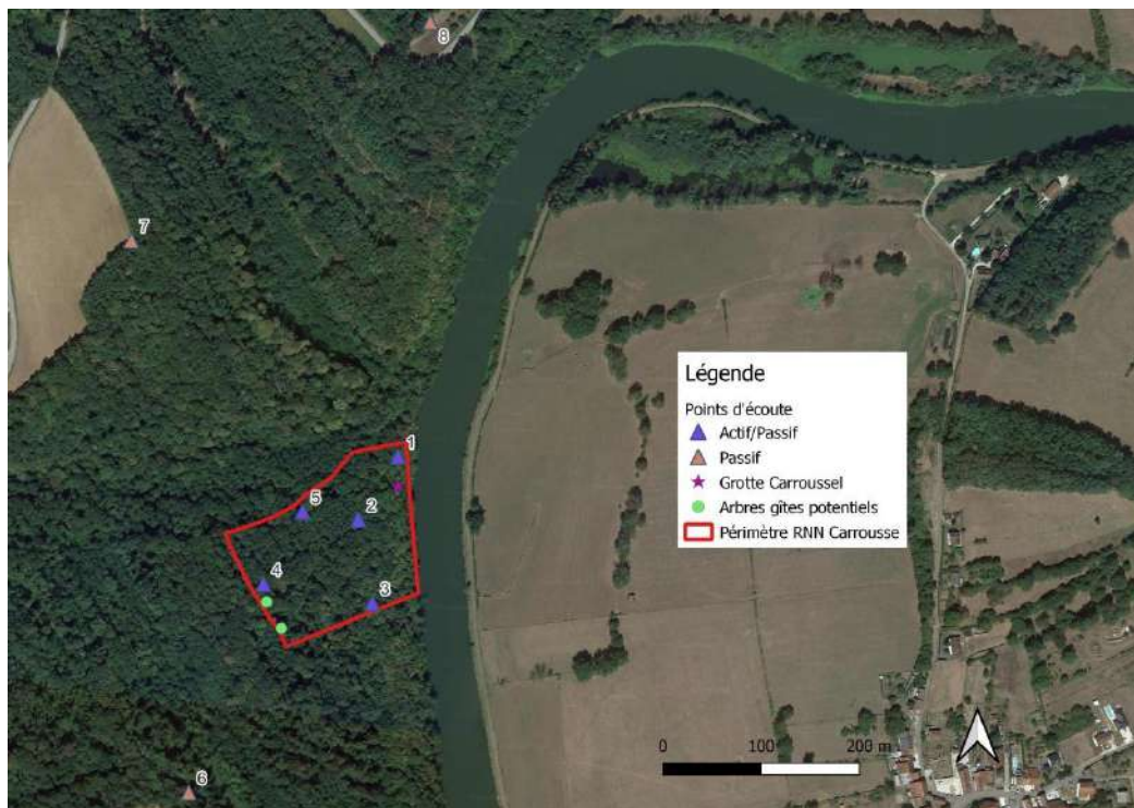
Figure 4 : Emplacement des arbres gîtes à cavités potentiels et points d'écoute de la RNN Grotte du Carroussel, CPEPESC FC 2024.
