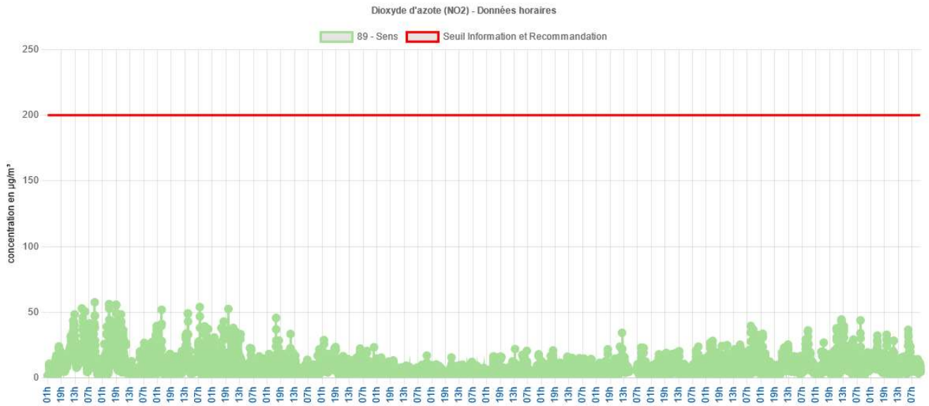
Modélisation des concentrations de dioxyde d'azote pour l'année 2024
