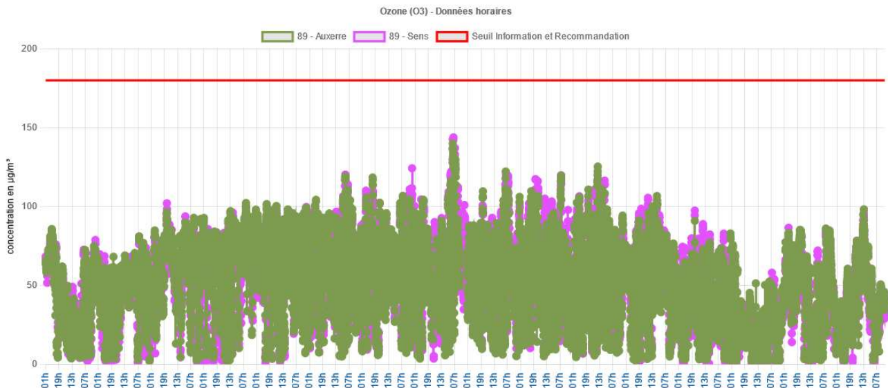
Modélisation des concentrations en ozone pour l'année 2024
