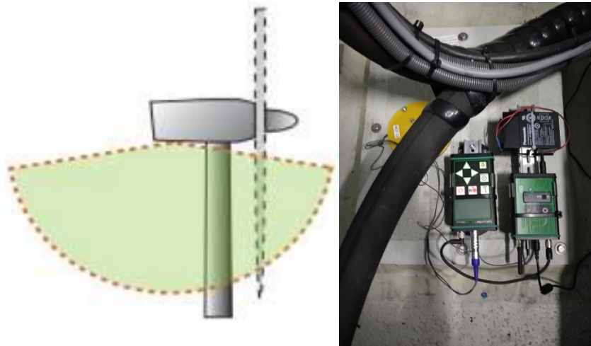
Figure 2: Matériel utilisé pour les écoutes en nacelle (Silva Environnement, 2018)
