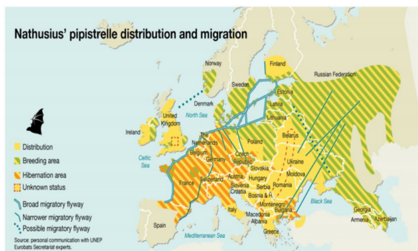
Figure 9: Routes migratoires de la Pipistrelle de Nathusius
