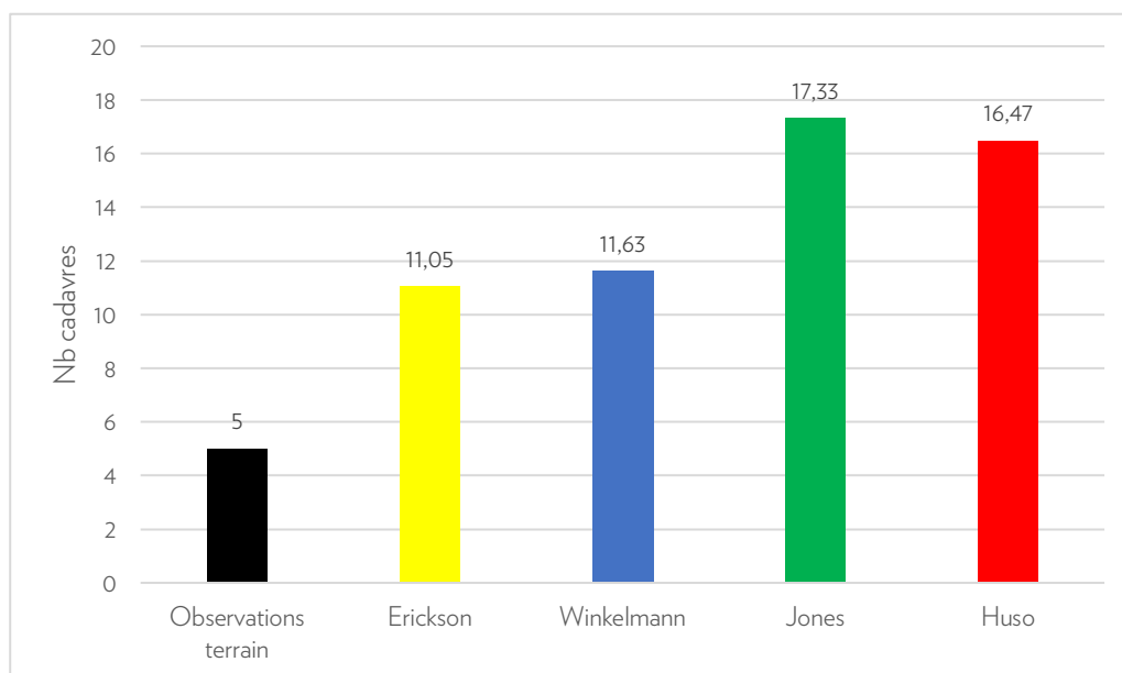
Figure 22: Estimation de la mortalité sur chaque éolienne en fonction des différents protocoles utilisés (nombre de chauves-souris tuées par an sur l'ensemble du parc de Bois des Saulx)
