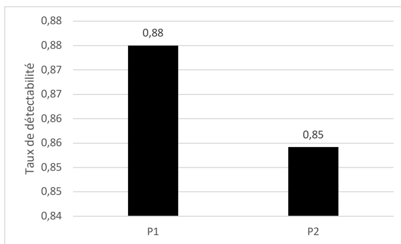
Figure 19: Résultats des tests d'efficacité de l'observateur
