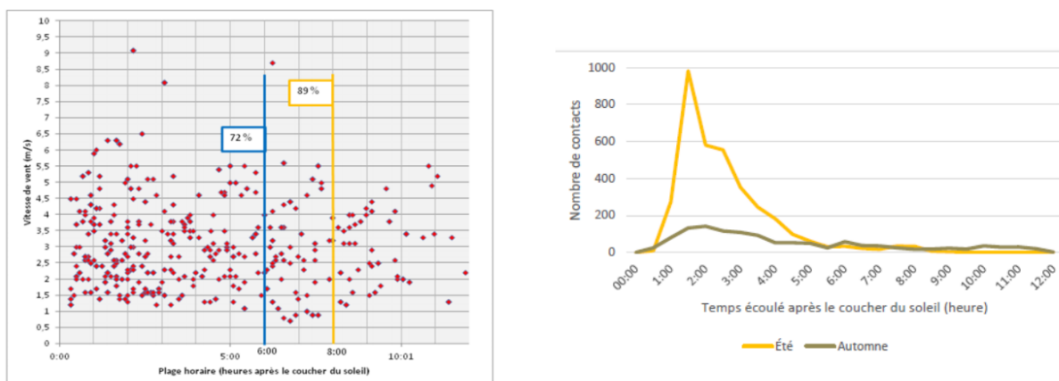
Figure 13: Distribution des contacts en fonction de l'heure de la nuit (Thauront et al., 2015 et Encis Environnement, 2015)
