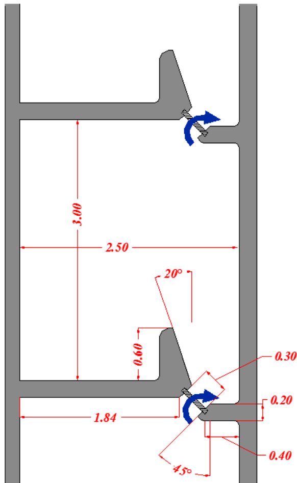
Fig. 31. Détail des caractéristiques géométriques d'un bassin
