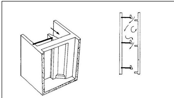
Fig. 24. Passes à fentes verticales (d'après LARINIER, 1992)
