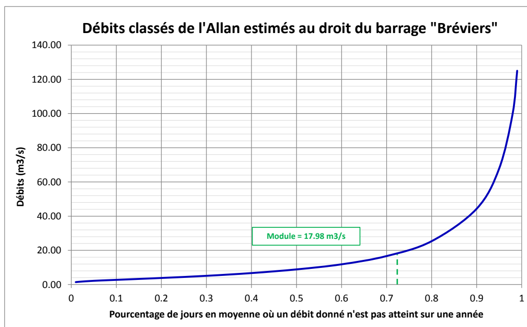
Fig. 11. Courbe des débits classés
