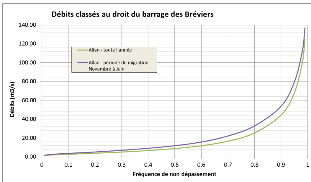
Fig. 18. Courbes de débits classés sur les plages de fonctionnement retenues
