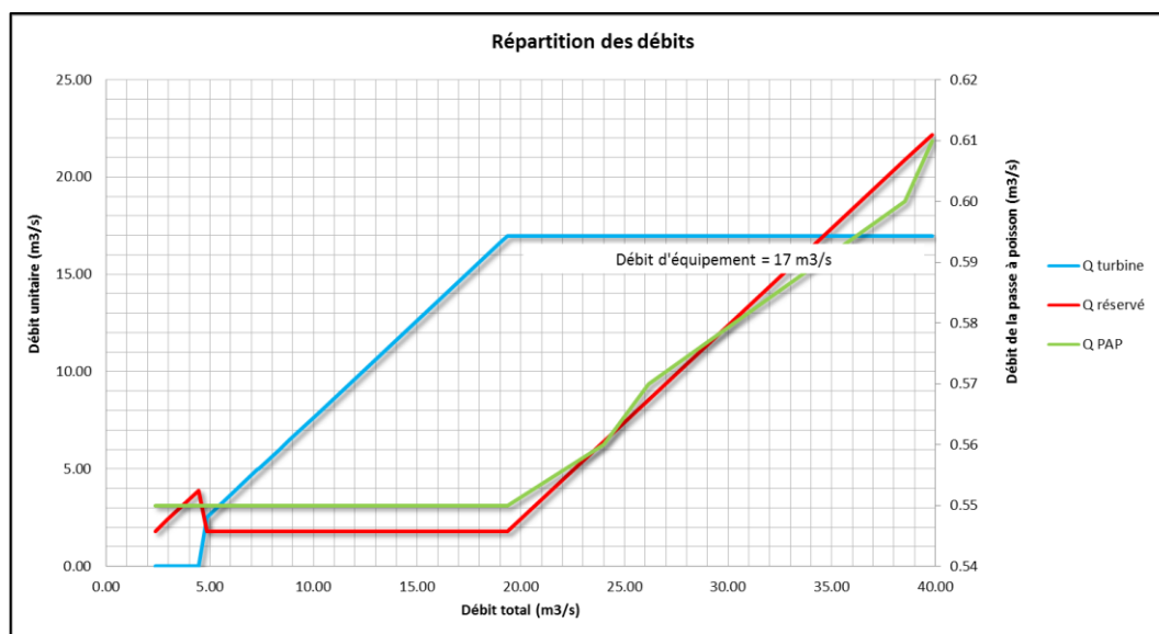
Fig. 28. Répartition des débits – Etat projet
