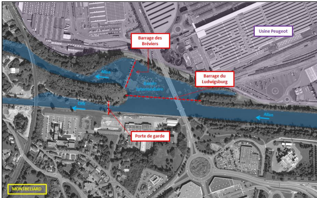
Fig. 2. Localisation du complexe hydraulique Ludwigsburg/Bréviers
