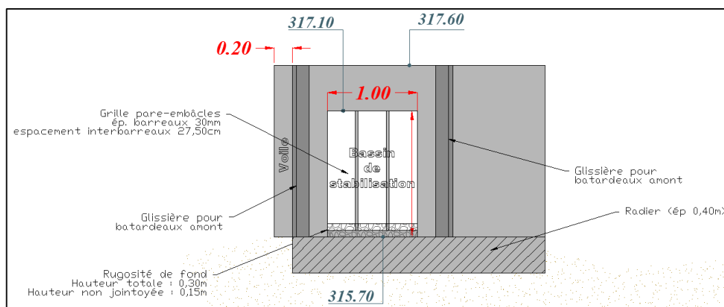
Fig. 32. Pare-embâcle situé en amont du bassin de stabilisation
