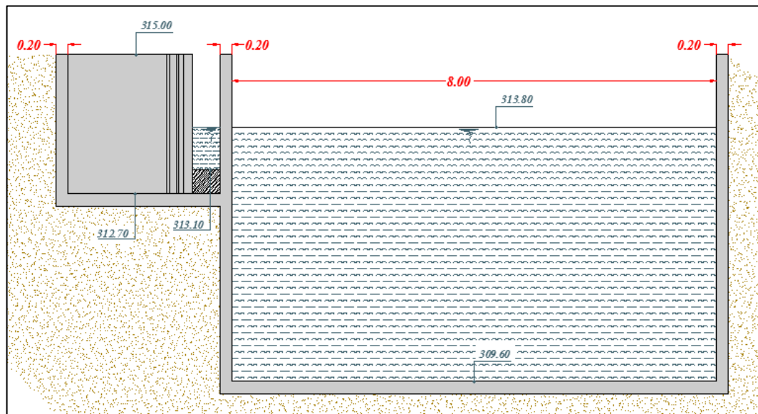
Fig. 27. Entrée de la passe piscicole – fente 45 cm
