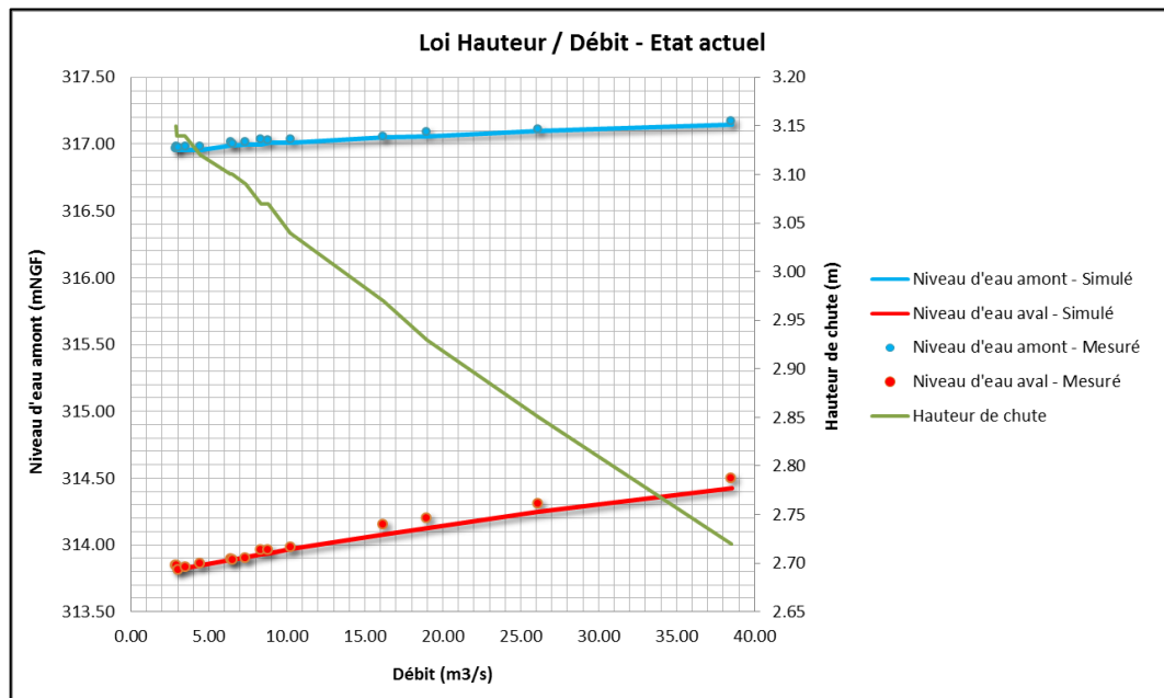
Fig. 12. Loi hauteur / débit de l'état actuel (modèle)
