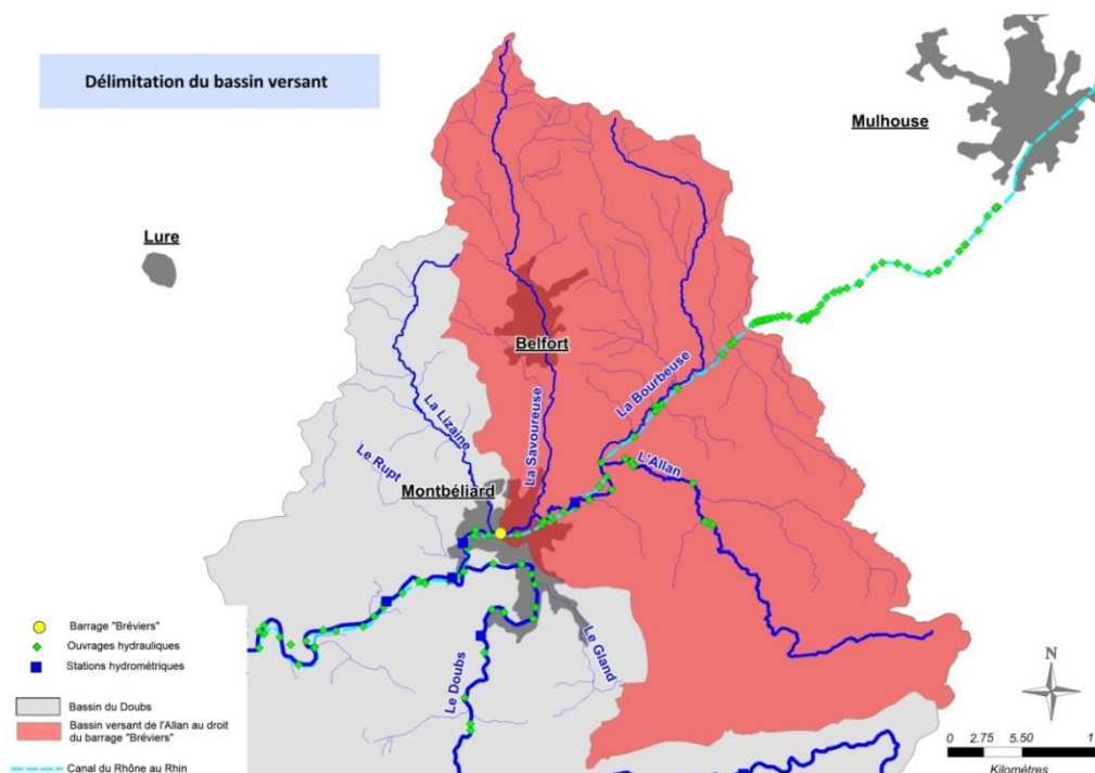
Fig. 1. Bassin versant de l'Allan drainé au droit du barrage « Ludwigsburg »
