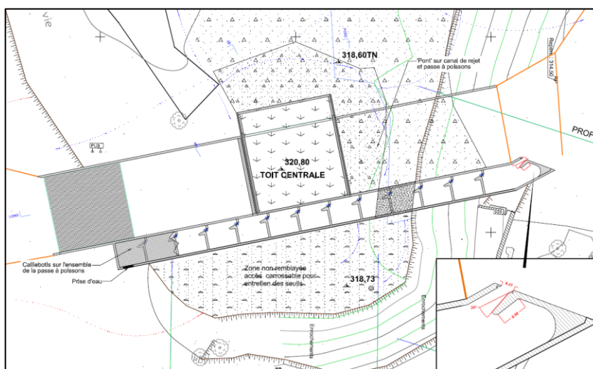
Fig. 26. Implantation de l'ouvrage
