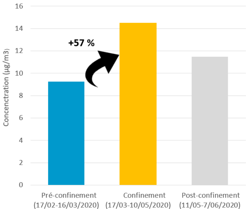
Evolution des niveaux en PM10 du 17/02 au 7/06/2020 Station de Vesoul
