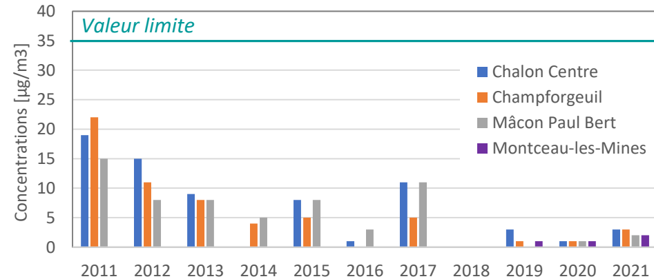
Nombre de dépassements de la valeur limite 50 \mu\text{g}/\text{m}^3 /jour en PM10 observés sur le département
