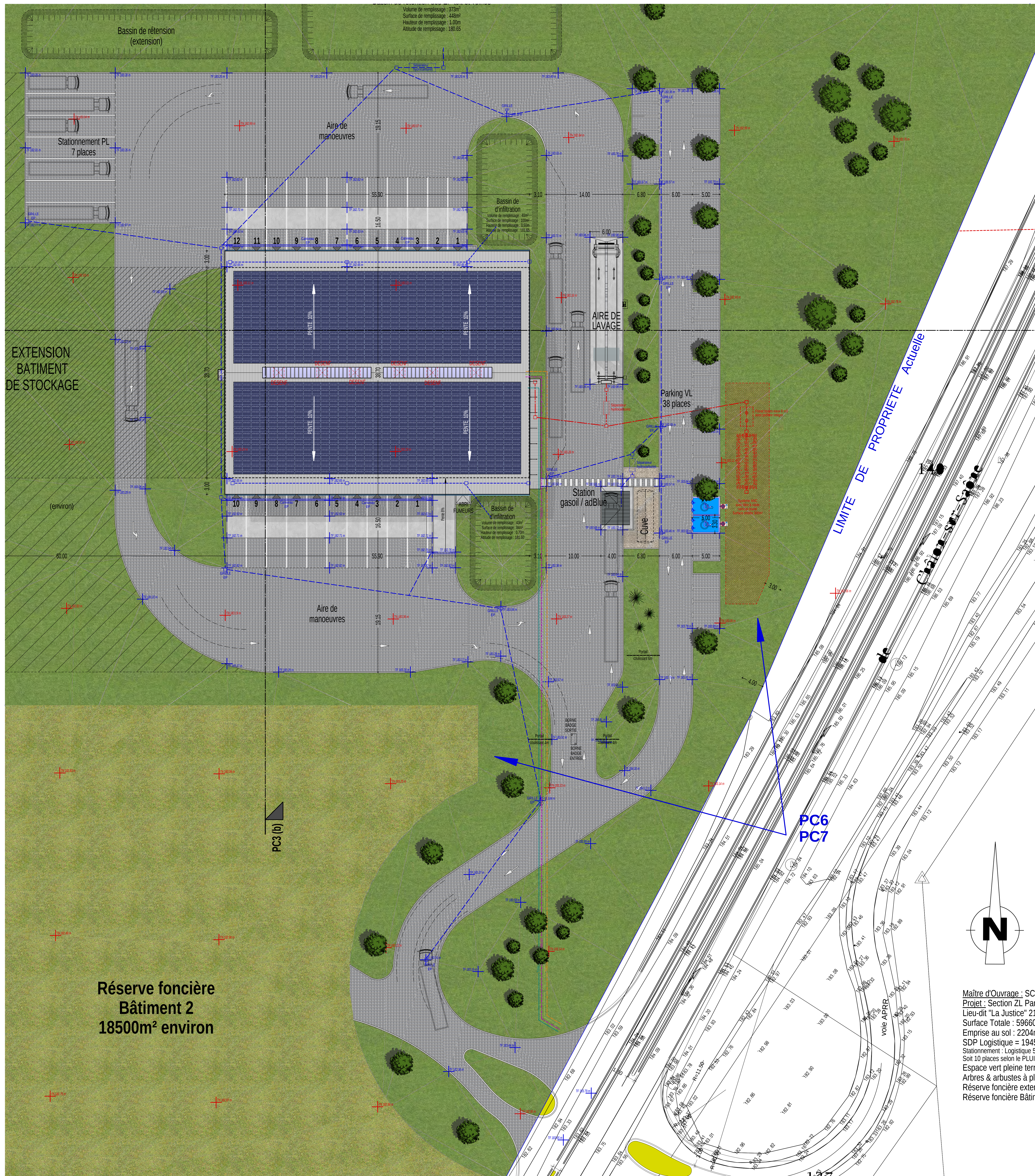
PC 2 - Plan de masse (extrait) Ech : 1/250eme
