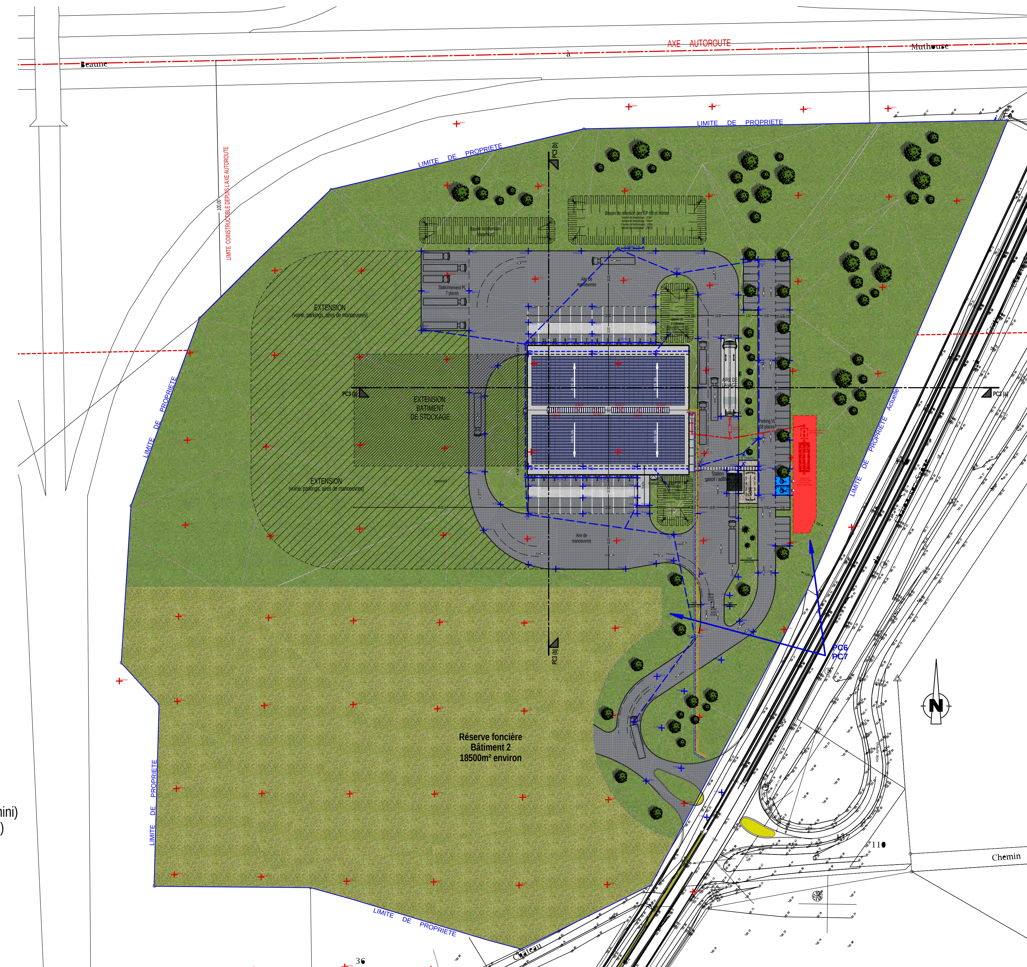
PC 2 - Plan de masse Ech : 1/750eme
