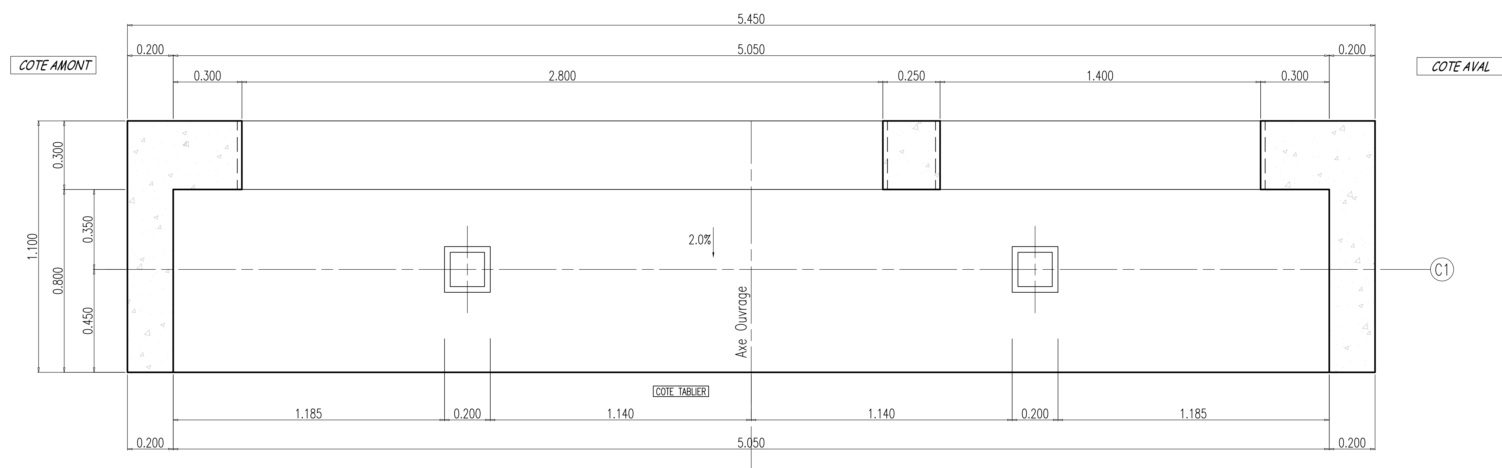
VUE EN PLAN CULEE 1/10
