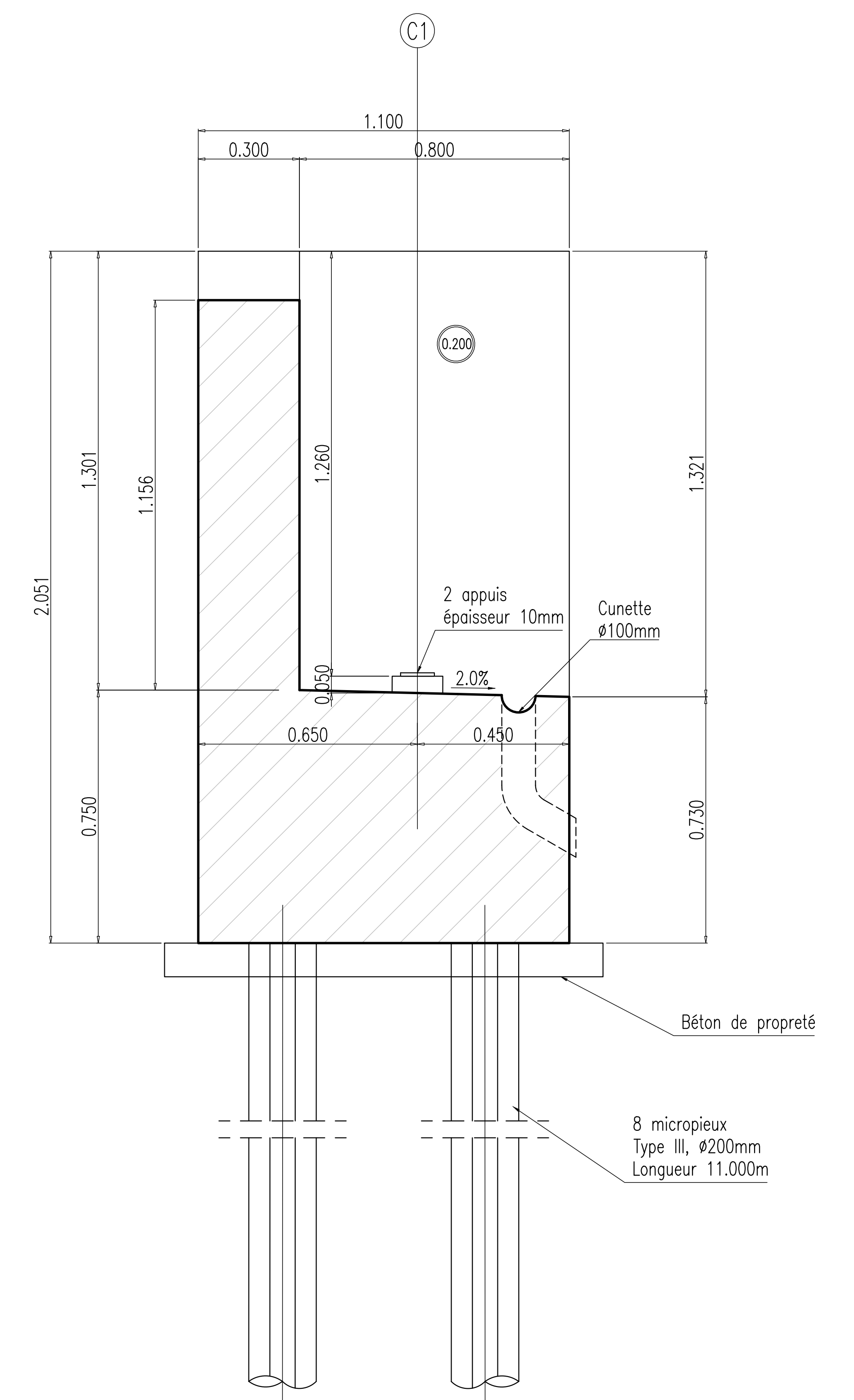
COFFRAGE CULEE COUPE TYPE 1/10
