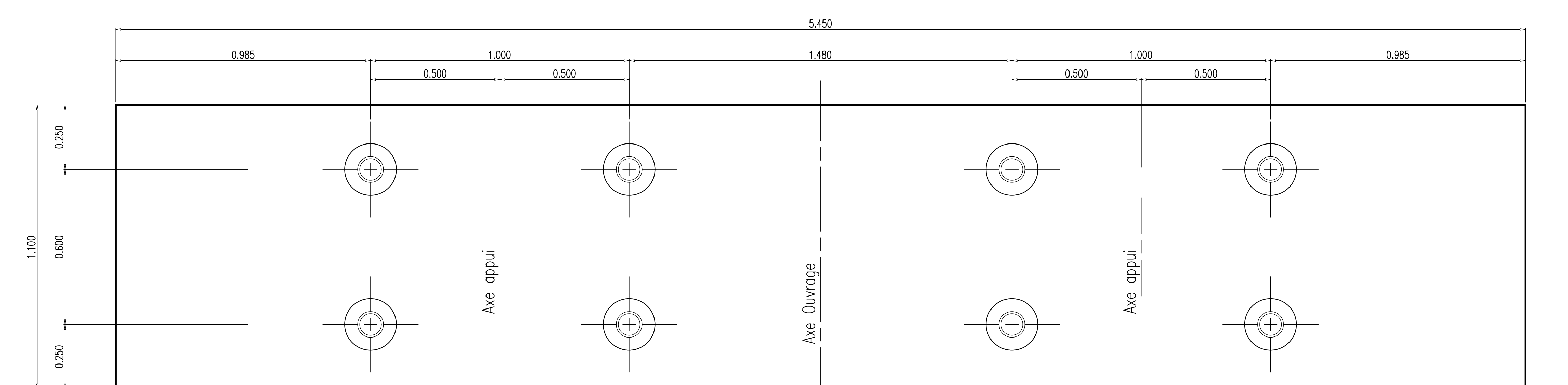
IMPLANTATION MICROPIEUX 1/10
