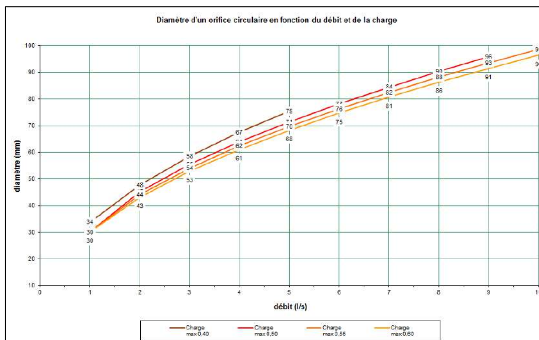
Figure 21 : Diamètre d'un orifice circulaire en fonction du débit et de la charge - Source : Ajutage Bordeaux-Métropole
