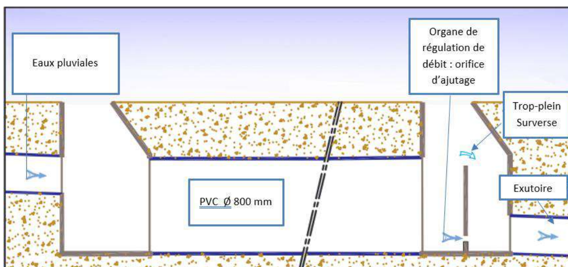
Figure 19 : Schématisation de la canalisation surdimensionnée
