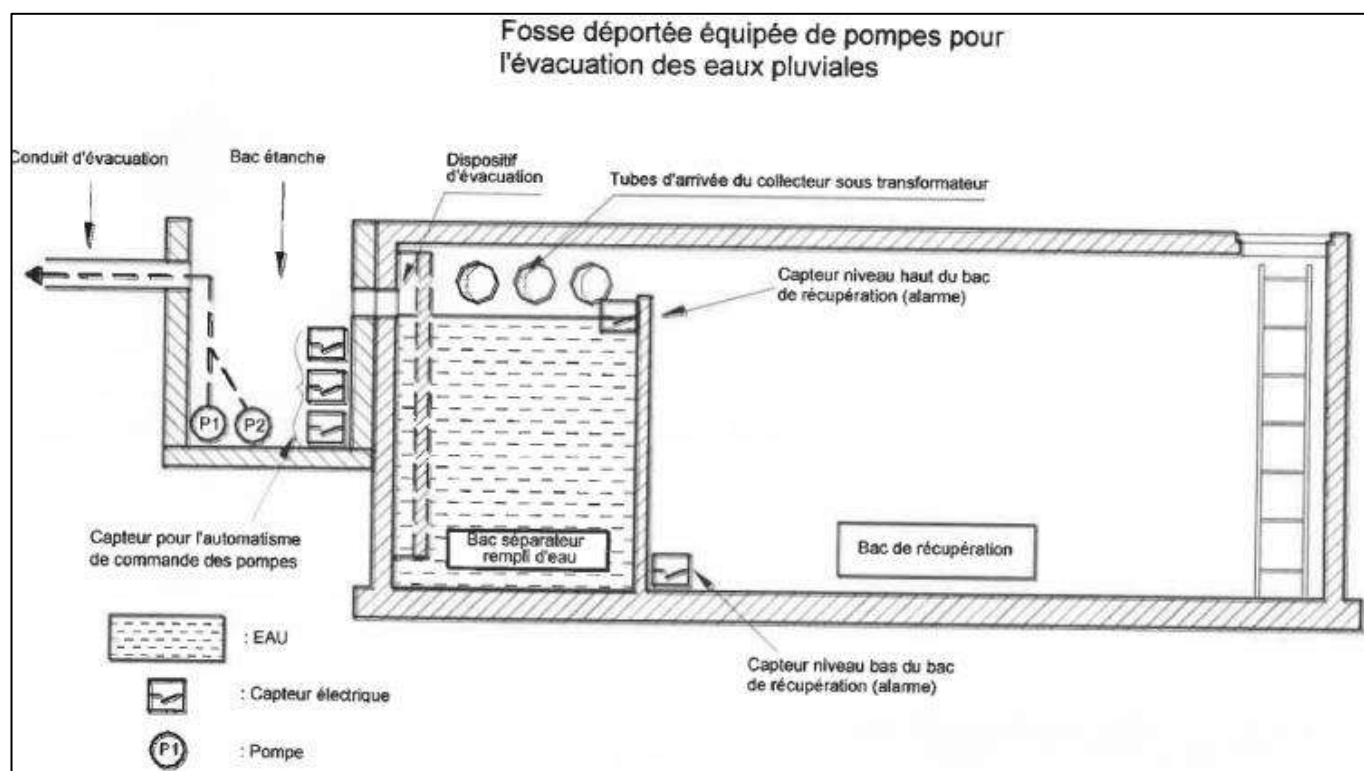
Figure 22 : Schéma de principe de la fosse déportée et capteur de niveau
