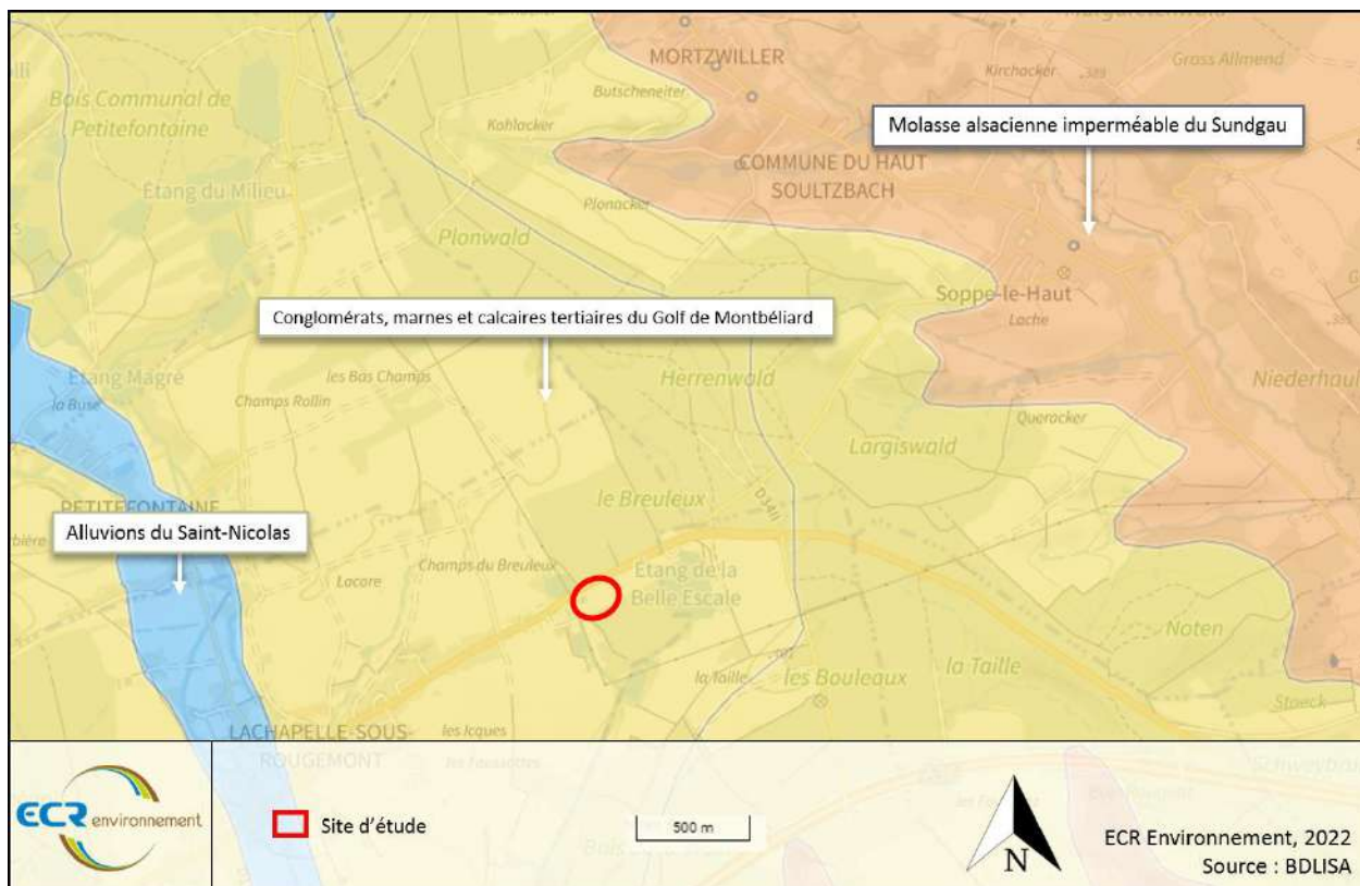
Figure 11 : Délimitation géographique de l'aquifère – BDLISA
