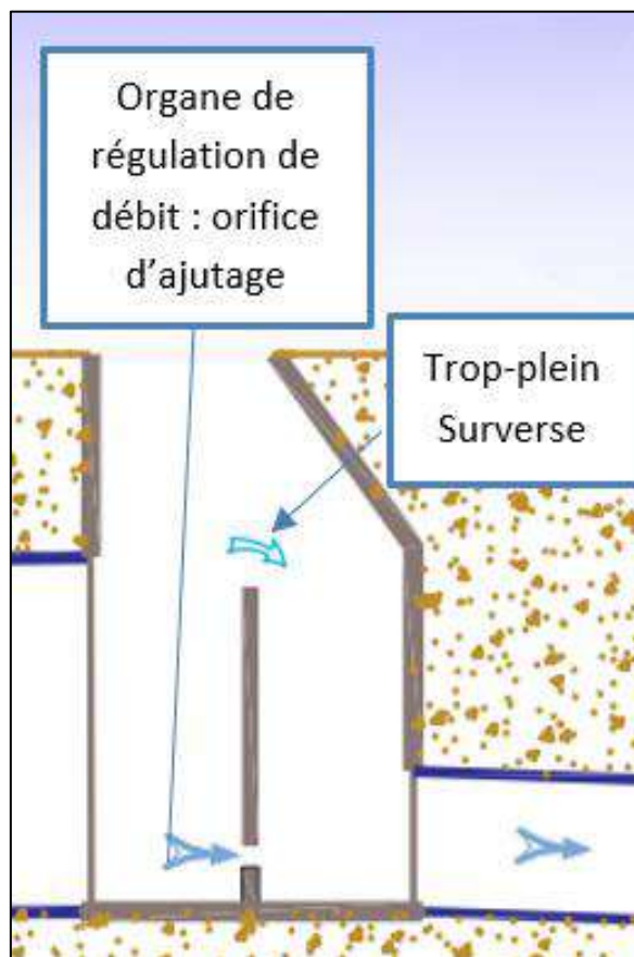
Figure 20 : Schéma de la coupe-type d'un organe de régulation de débit : orifice d'ajutage
