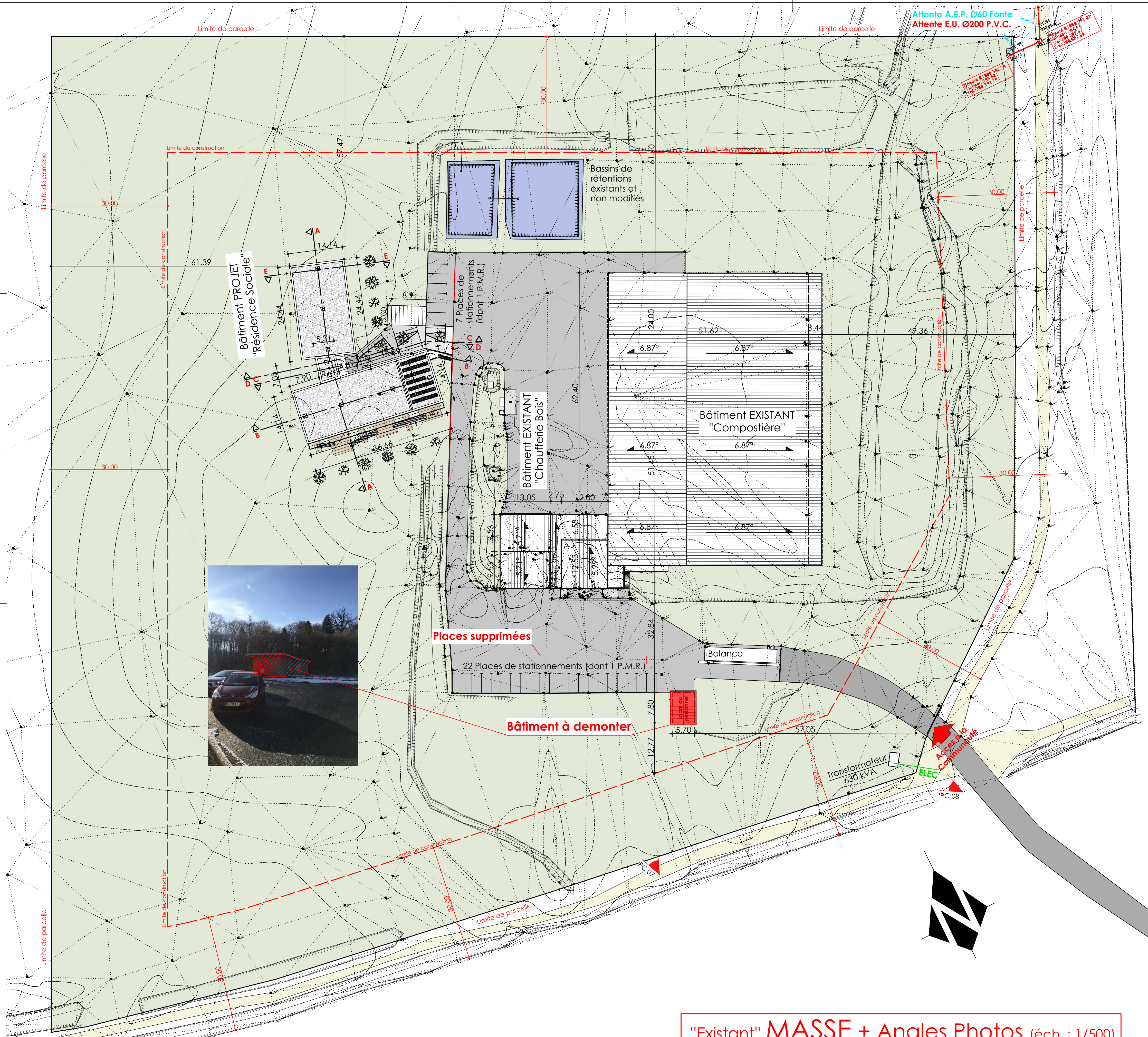
"Existant" MASSE + Angles Photos (éch. : 1/500)
