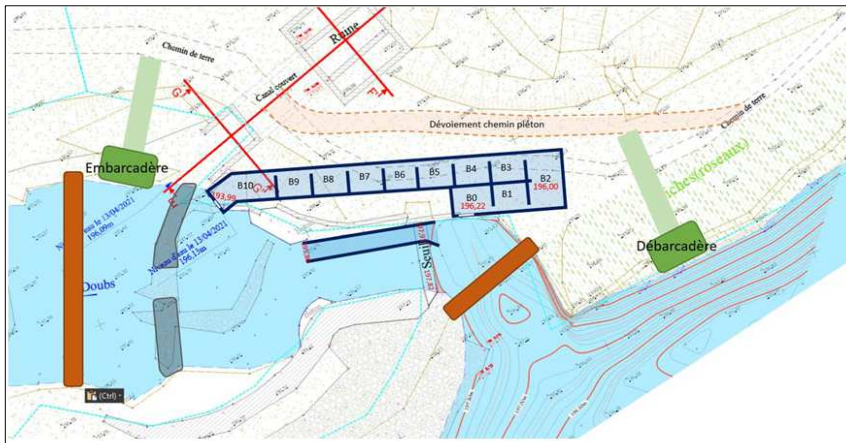
Plan d'implantation de la future passe à poissons
