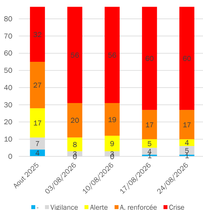
Evolution des niveaux d'étiage aux stations
