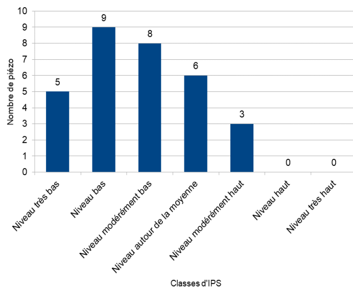
Indicateur Piézométrique Standardisé
