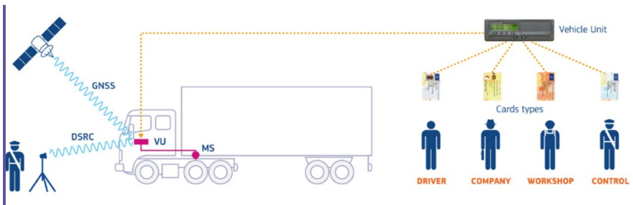
Le chronotachygraphe intelligent et ses composants
