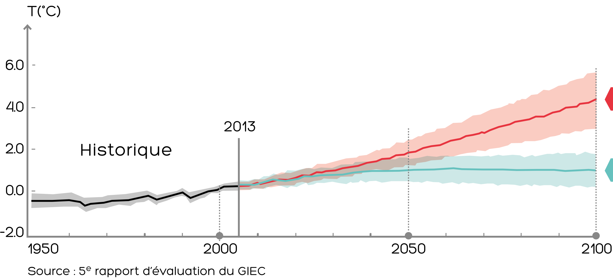
ÉVOLUTION DE L'ANOMALIE DE TEMPÉRATURE MOYENNE DU GLOBE, EN SURFACE, DE 1950 À 2100, SIMULÉE PAR L'ENSEMBLE DES MODÈLES DE CLIMAT POUR DIFFÉRENTES FAMILLES DE SCÉNARIOS D'ÉMISSIONS.
