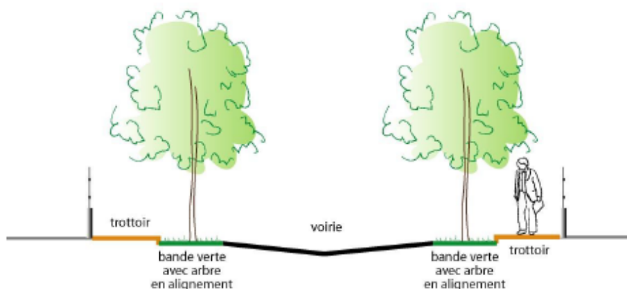
Profils en « V » des voies permettant un stockage provisoire des eaux
